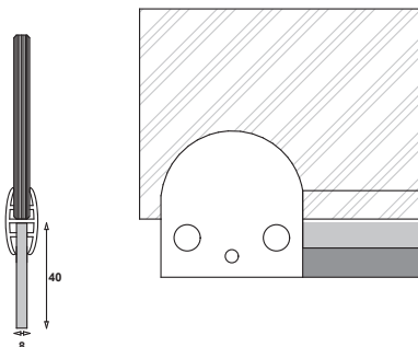
Infinia 211, 214, Vetro 511, 514 asennus tiivistesokkelin kanssa
