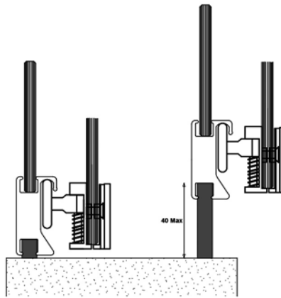
Infinia 300 ja 400 -sarjat Asennus sokkelin päälle
